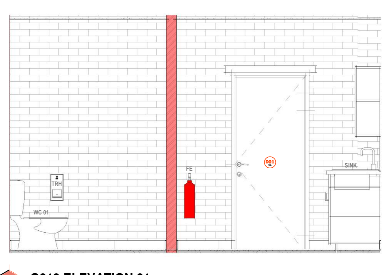
G019 ELEVATION 01 1:25
