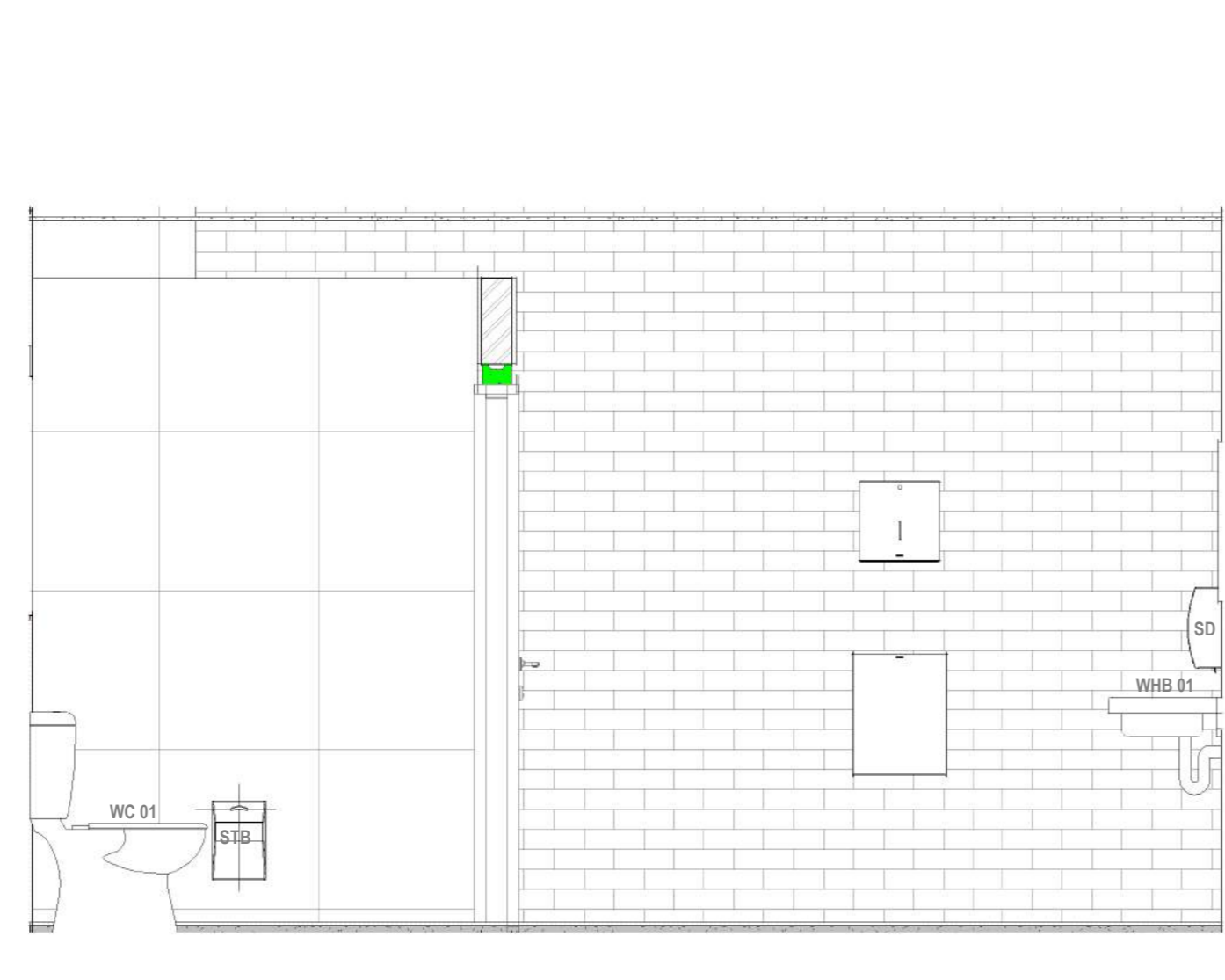
G012 ELEVATION 01 1:25
