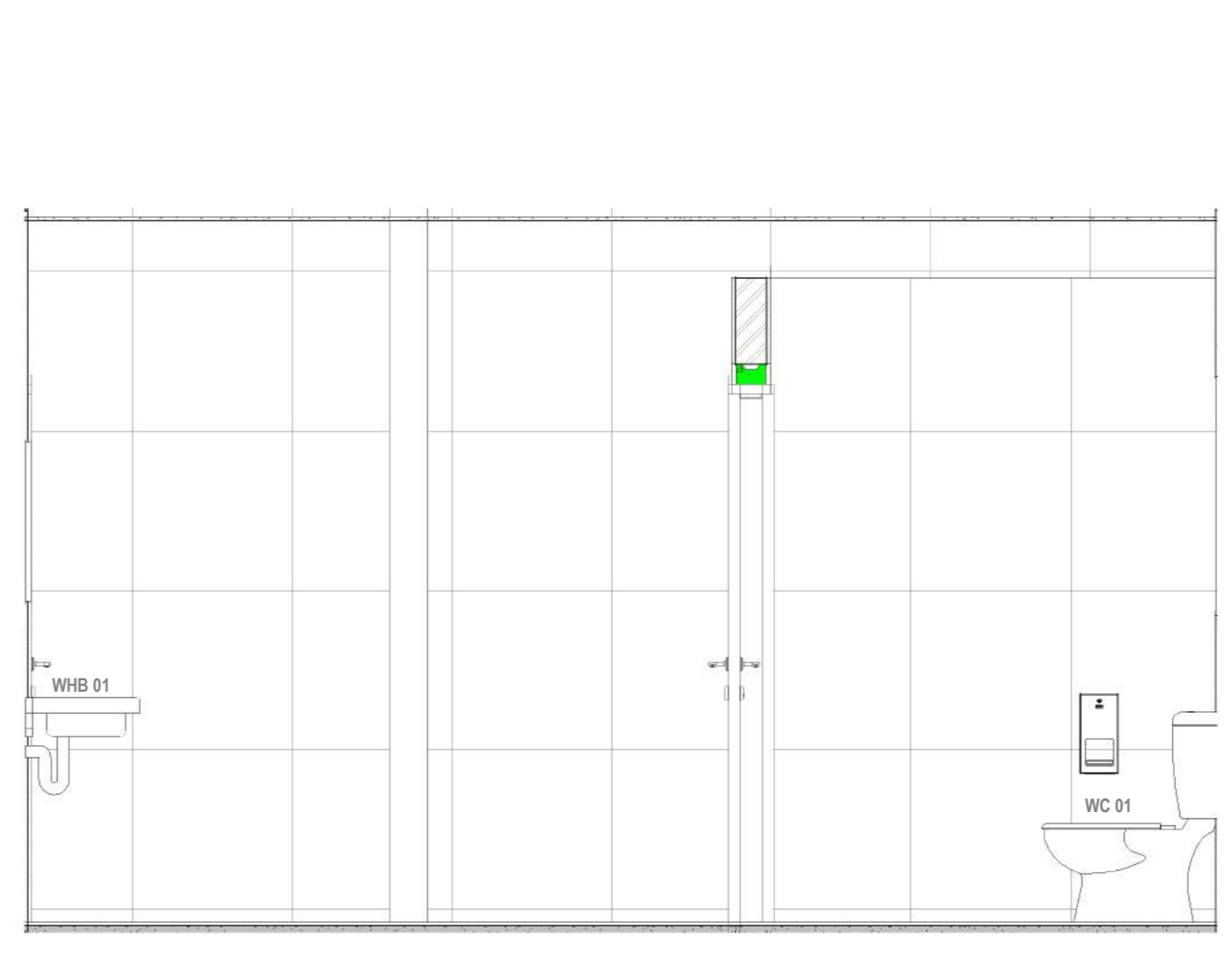
G012 ELEVATION 03 1:25
