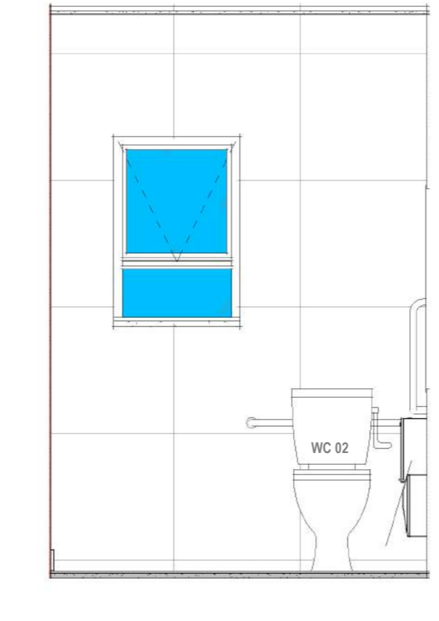
G014 ELEVATION 02 1:25
