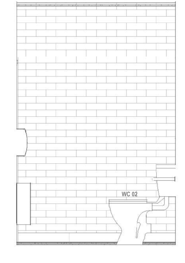
G014 ELEVATION 01 1:25
