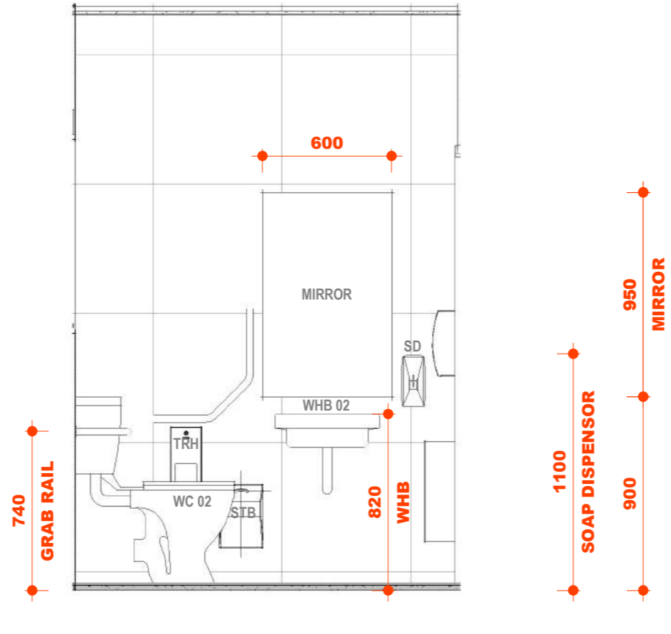
G014 ELEVATION 03 1:25
