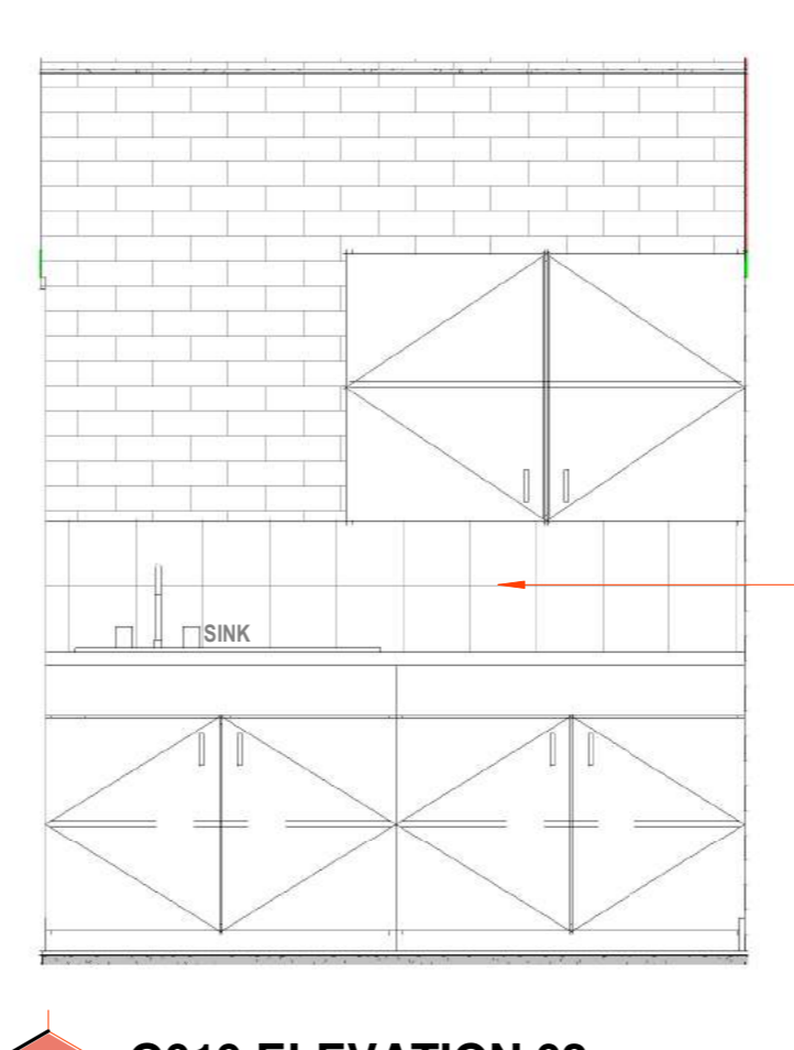
G019 ELEVATION 02 1:25
