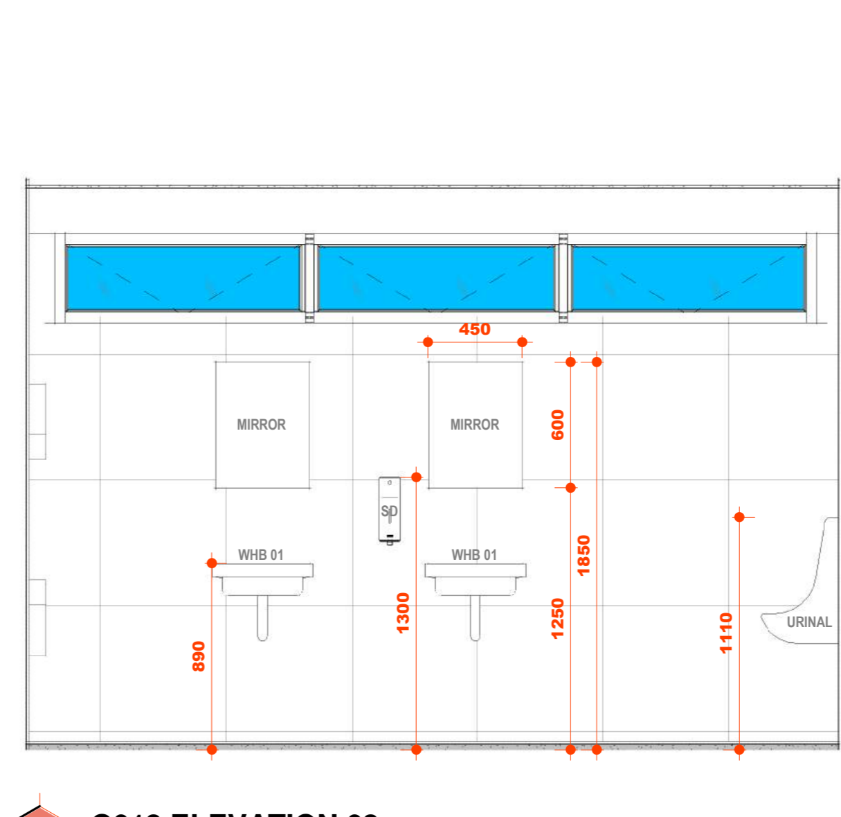
G012 ELEVATION 03 1:25
