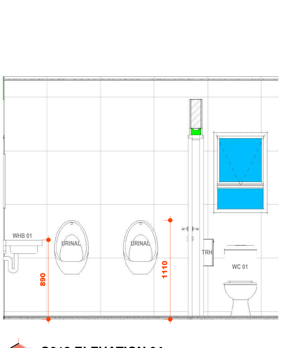
G012 ELEVATION 04 1:25
