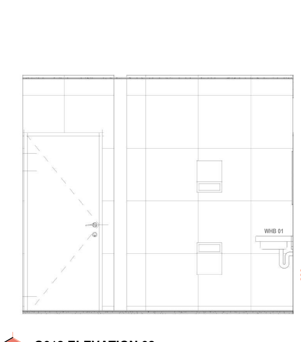
G012 ELEVATION 02 1:25
