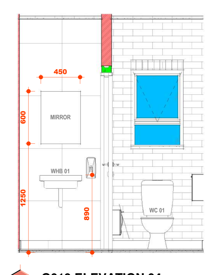
G019 ELEVATION 04 1:25
