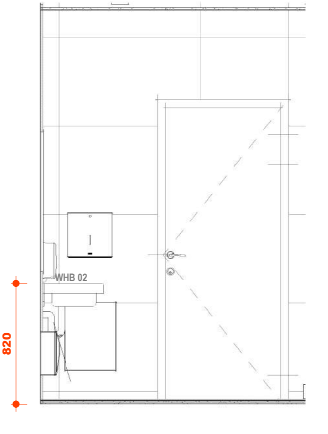
G014 ELEVATION 04 1:25
